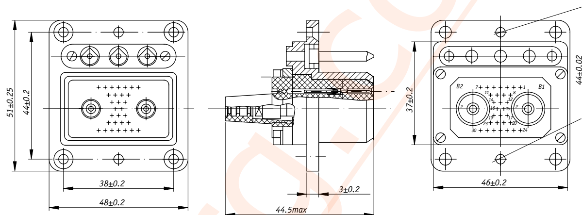
Рисунок 11 - Кабельная часть одинарного соединителя ОКП-BS-68
