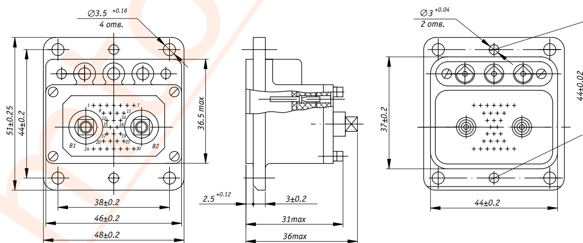
Рисунок 12 - Приборная часть одинарного соединителя ОКП-BS-68
