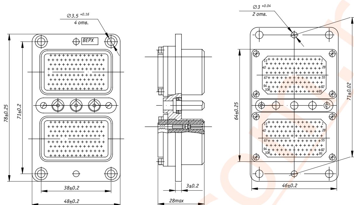
Рисунок 5 - Кабельная часть сдвоенного соединителя ОНП-ВС-54
