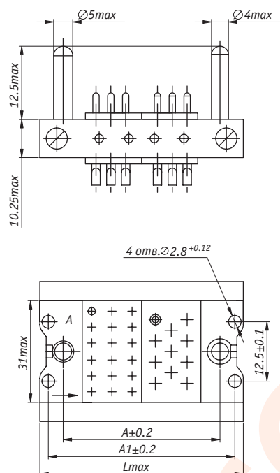
Рисунок 5 - Вилка приборная без кожуха, предназначенная для сочленения с блочной розеткой
