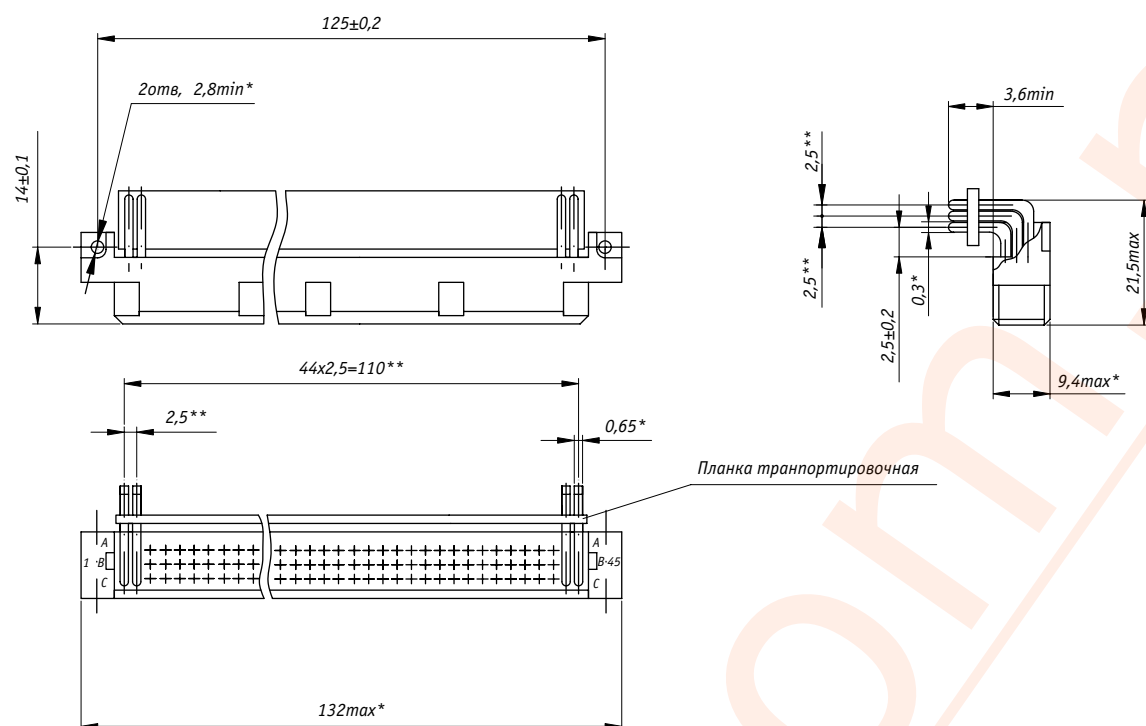
Рисунок 3 - Розетка
