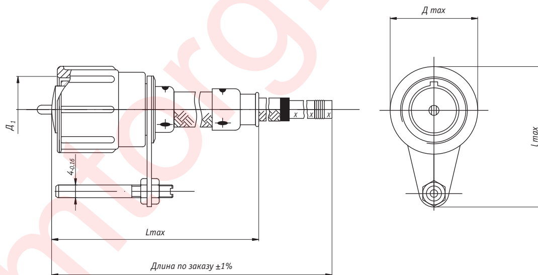
Рисунок 3 - Кабельная вилка
