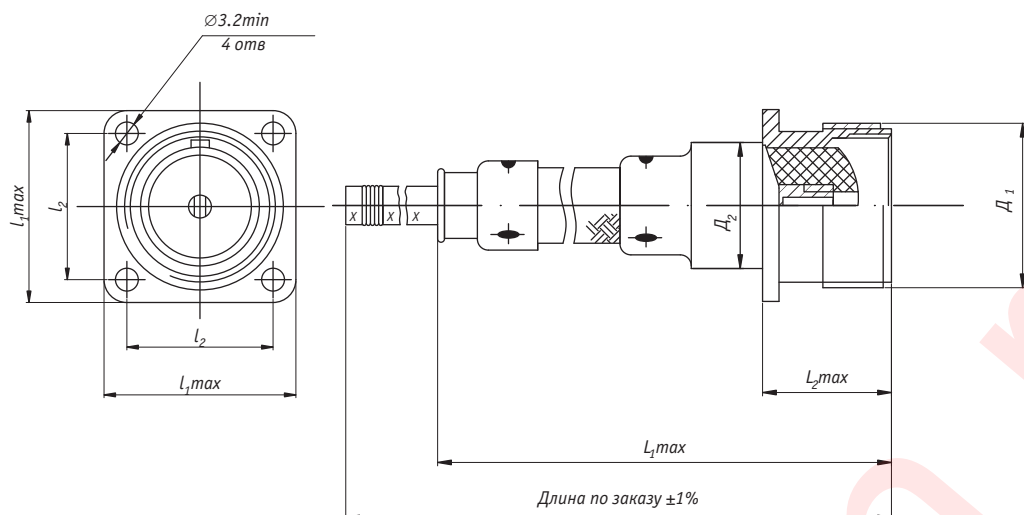
Рисунок 2 - Блочная розетка
