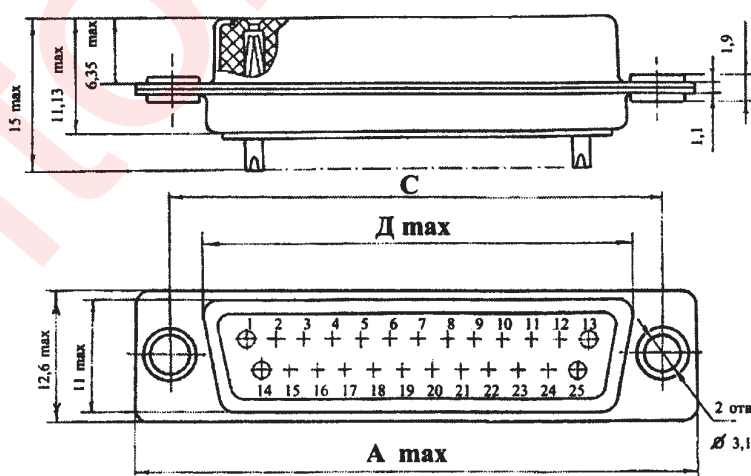
Рисунок 1 - Вилка (розетка) объемного монтажа
