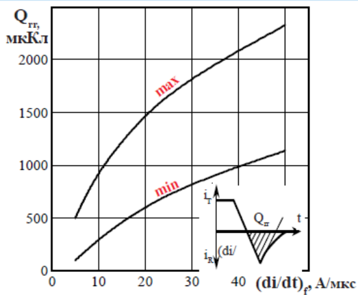
Рисунок 10 - Зависимость заряда восстановления Q_{\pi} от скорости спада тока (di/dt)_f в открытом состоянии при T_{jm} = 140^{\circ}\text{C} ; U_R = 100\text{ В} ; I_1 = I_{TAVM} .
