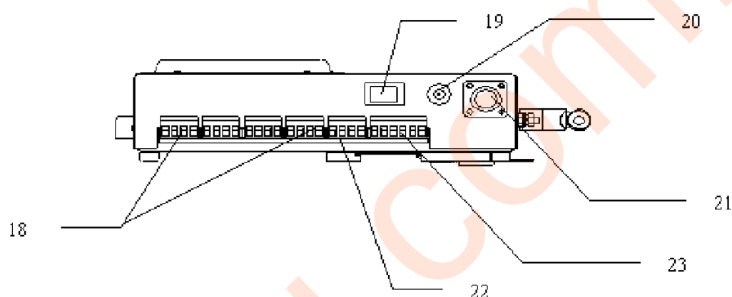
Рисунок 4 – ВИЗИР-5, вид сбоку (справа)
